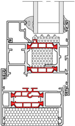
58BW CASEMENT HI JAMB
