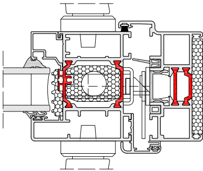
BSF70 HI LOCKING JAMB
