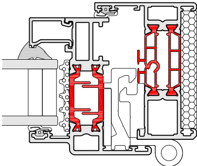
HERITAGE DOOR OPEN OUT HINGE JAMB
